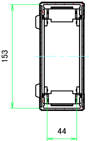
A-A ( 1:3.5 )
